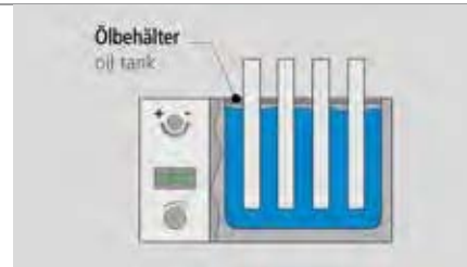
Temperaturprüfungen nach Flexa Norm 1034 Temperature tests acc. to Flexa norm 1034
